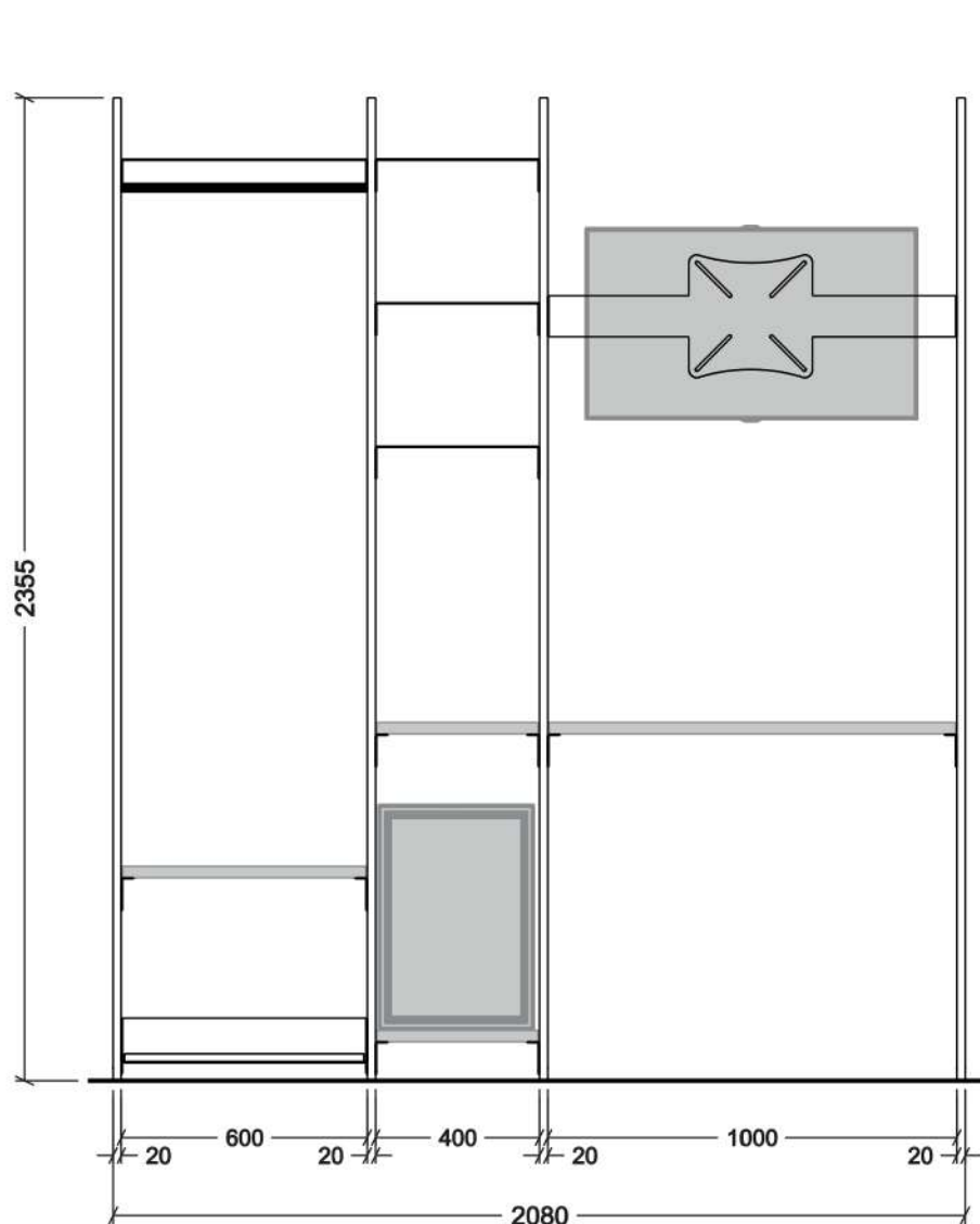
PROSPETTO FRONTALE
