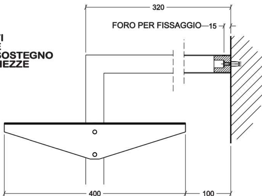
PARTICOLARE FISSAGGIO PARETE
