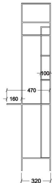
PROSPETTO LATERALE
