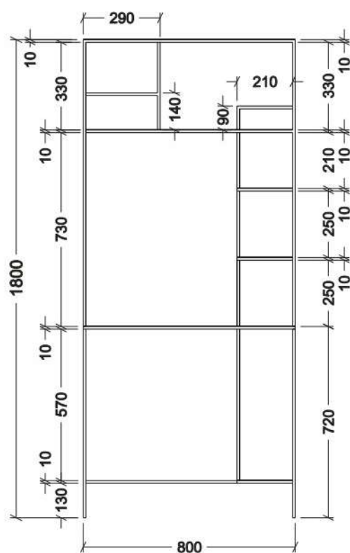
PROSPETTO FRONTALE
